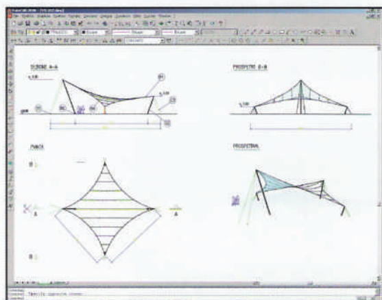
Progetto di una Tensostruttura a Vela .
